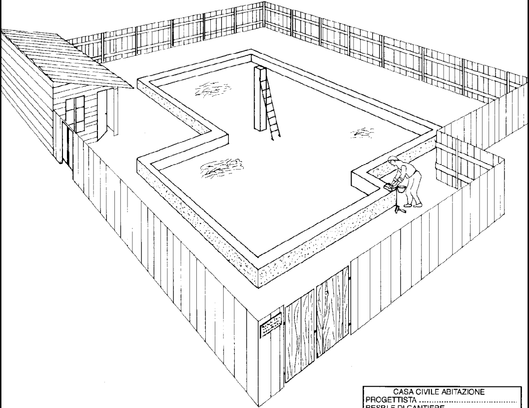
PROSPETTO-INGRESSO CANTIERE-
