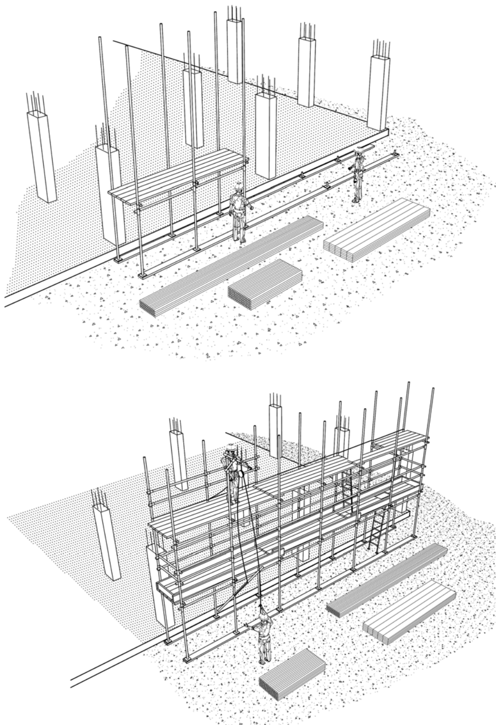
Fig.1 Ponteggio a tubo e giunto - montaggio primo e secondo piano
