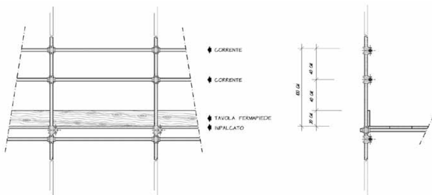
Parapetto di ponteggio a telaio prefabbricato
